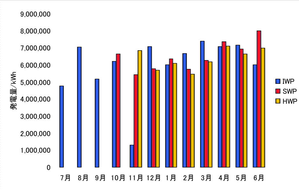
岩国WP・白河WP・日田WP 発電電力量推移
